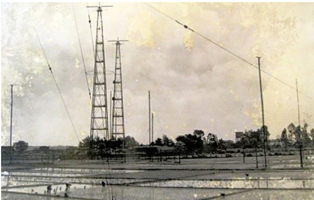
Das Antennensystem der Senderstation Me Tri während des Krieges. (Foto: VOV)
